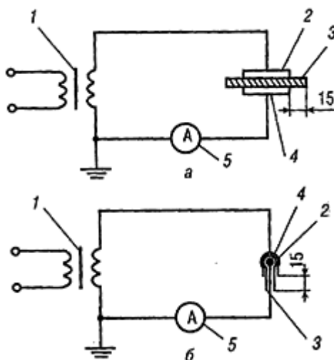
Рис.2.5. Схемы электрических испытаний гибкого изолирующего покрытия (а) и гибкой изолирующей накладки (б):
