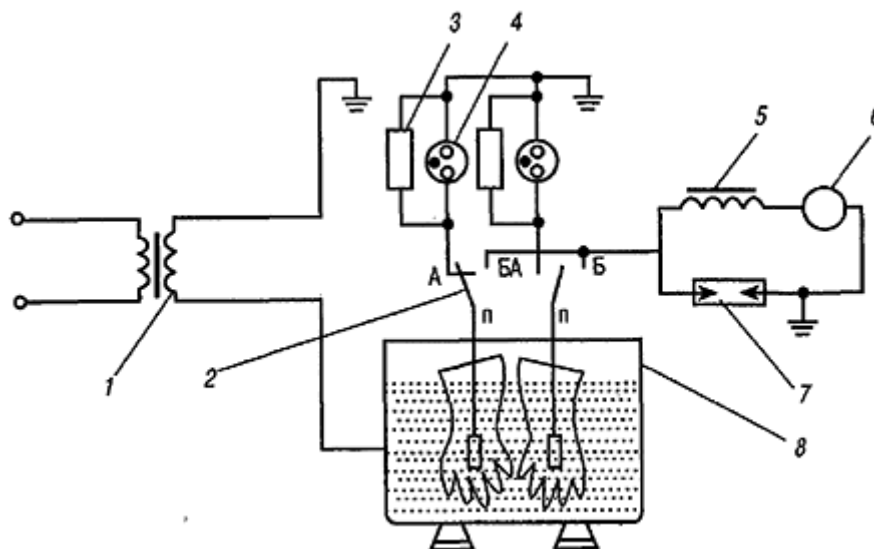
Рис.2.3. Принципиальная схема испытания диэлектрических перчаток, бот и галош: 1 - испытательный трансформатор; 2 - контакты переключающие; 3 - шунтирующее сопротивление (15-20 кОм); 4 - газоразрядная лампа; 5 - дроссель; 6 - миллиамперметр; 7 - разрядник; 8 - ванна с водой
